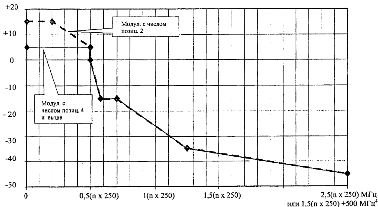
Рисунок 1. Маска спектра излучаемого сигнала
