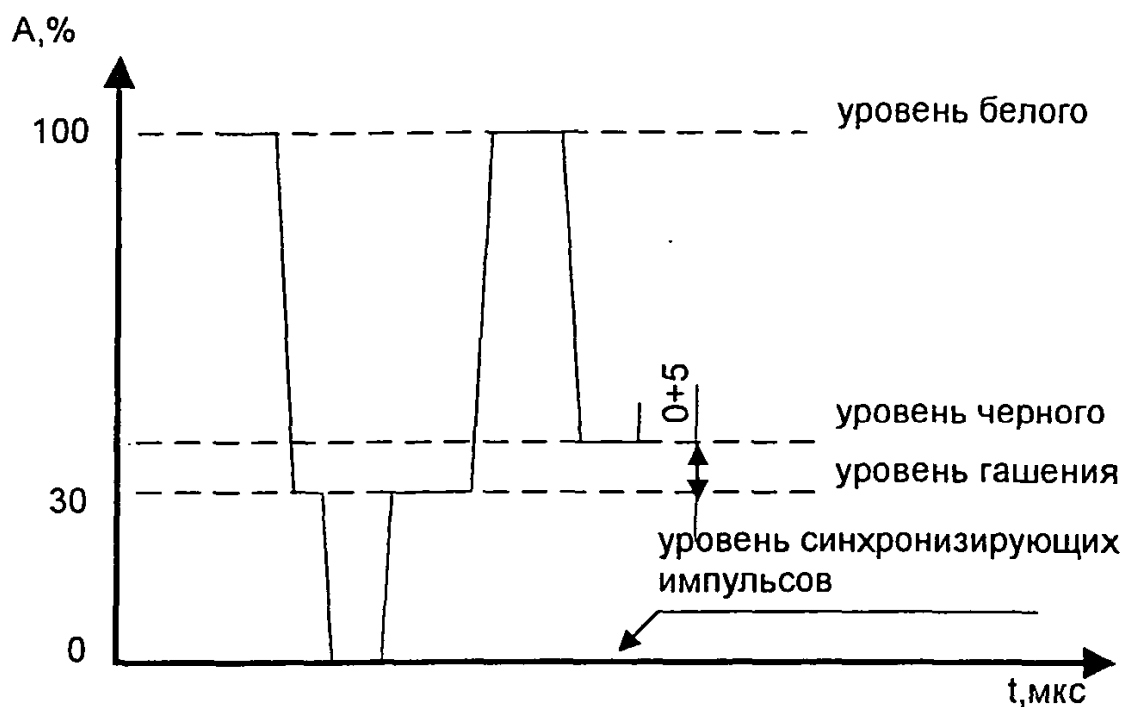
Рисунок П.2.1. Уровни входного видеосигнала
