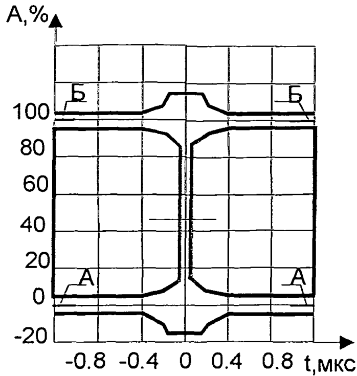
Рисунок П.2.3. Поле допуска переходной характеристики
