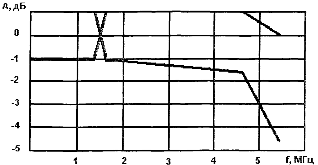
Рисунок П.2.3. Поле допуска переходной характеристики
