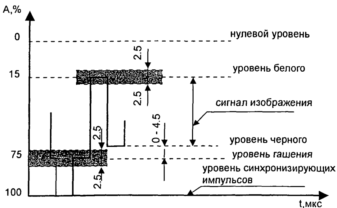
Рисунок П.2.2. Уровни выходного радиосигнала изображения
