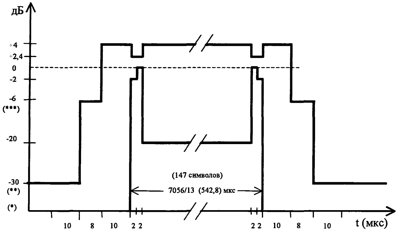
Рисунок 2. Маска при 8-ми позиционной фазовой модуляции
