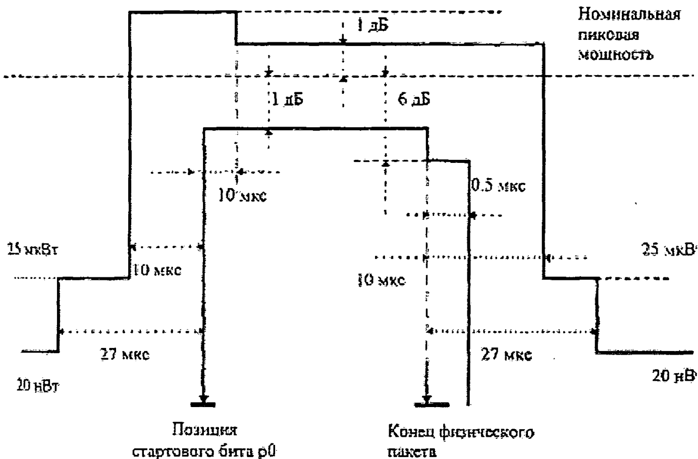
Рисунок 1. Шаблон огибающей передаваемого пакета
