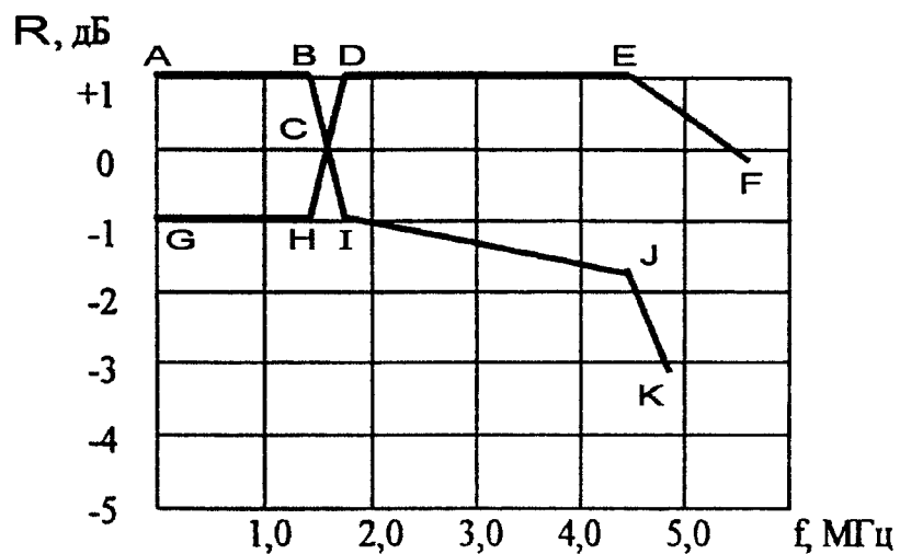
Рисунок 2. Шаблон допустимых значений сквозной АЧХ канала изображения по стандарту В/Г (PAL)
