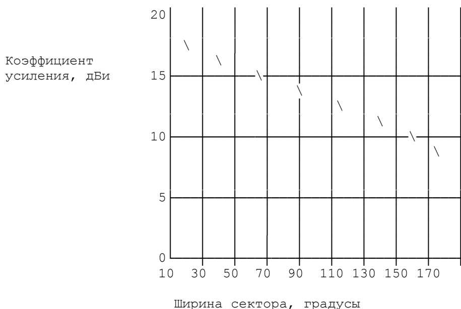
Рисунок 3. Значение коэффициента усиления для антенн базовой станции в диапазоне частот от 40,5 до 43,5 ГГц
