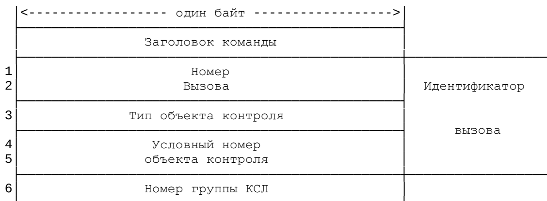
Рисунок 8. Формат команды N 7
