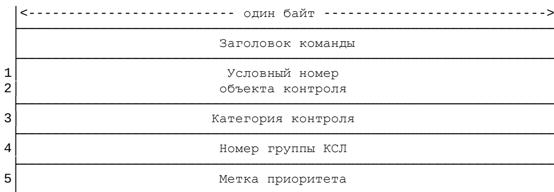
Рисунок 16. Формат команды N 15
