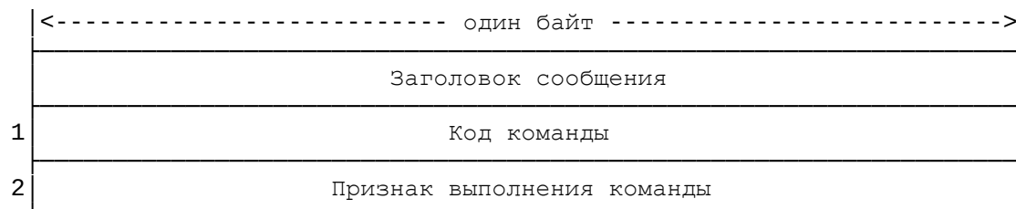
Рисунок 8. Формат сообщения N 8
