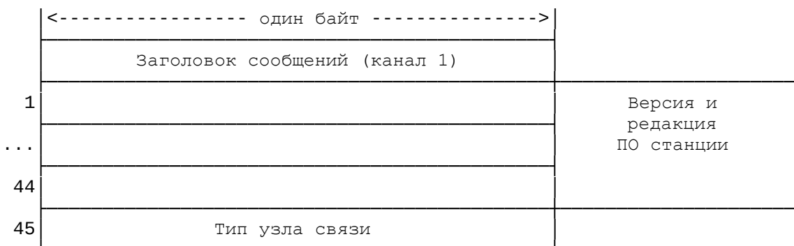
Рисунок 11. Формат сообщения N 11
