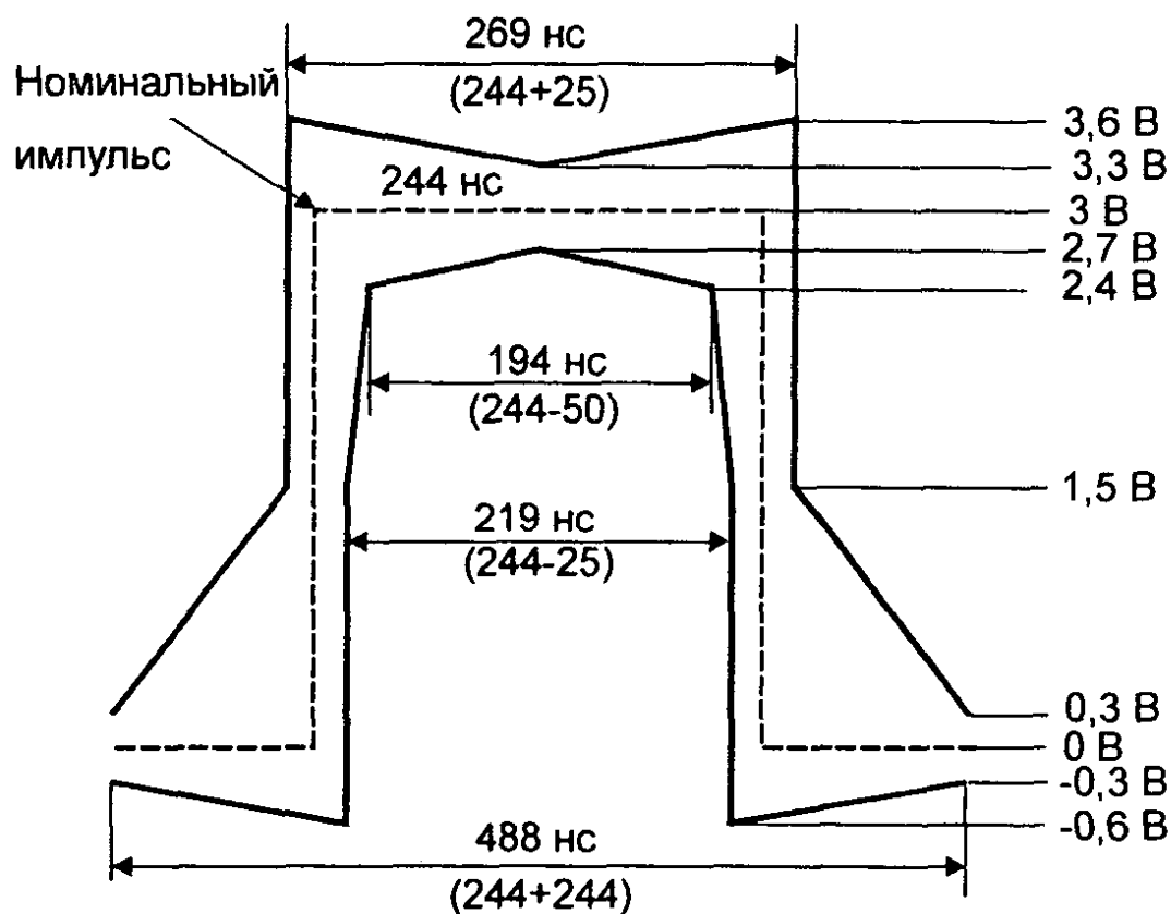
Рисунок 1. Маски импульса для интерфейса 2048 кбит/с
