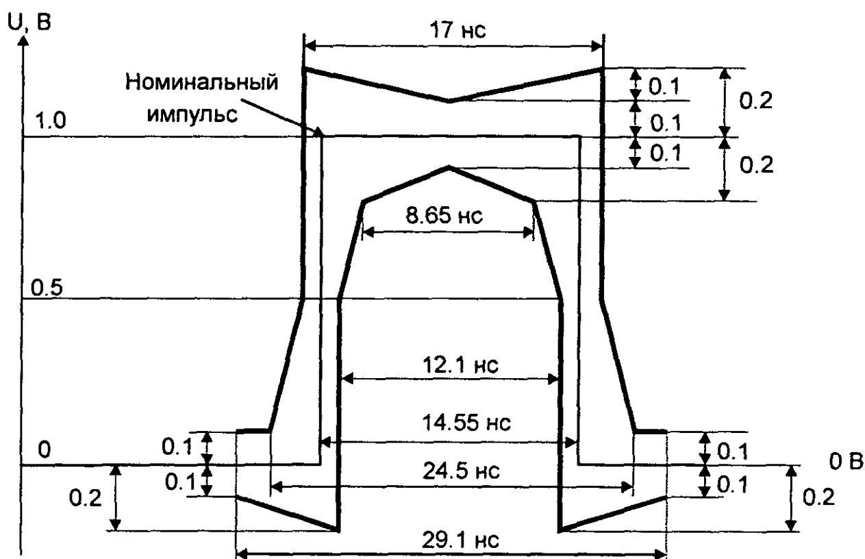
Рисунок 3. Маски импульса для интерфейса 34368 кбит/с
