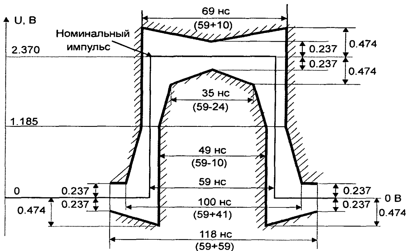
Рисунок 2. Маски импульса для интерфейса 8448 кбит/с
