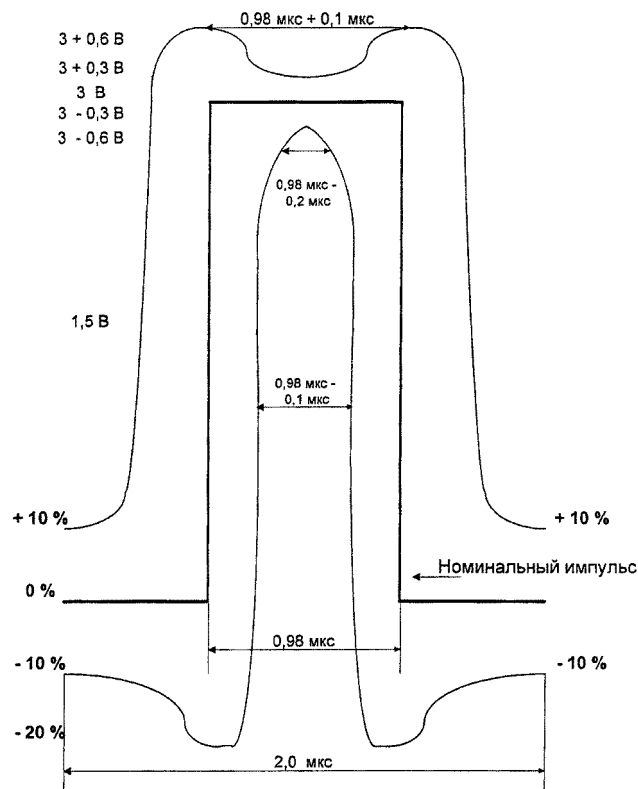
Рисунок. Шаблон импульса на стыке 1024 кбит/с
